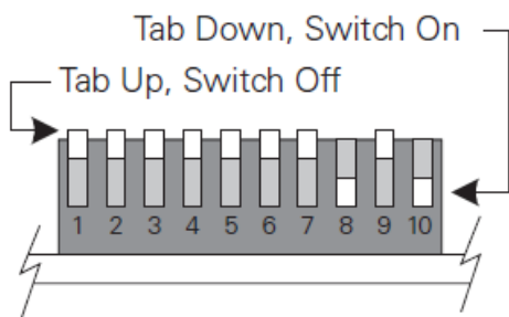
【図 3】ディップスイッチの番号とON/OFFの切換
