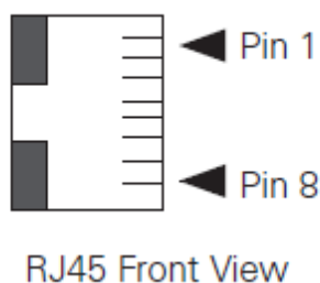
【図 13】 HS ポートのピン番号
