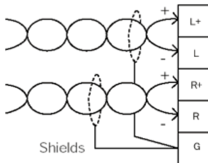
バランスステレオ音声の結線
