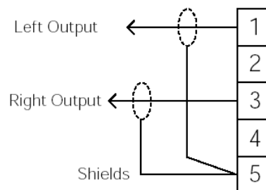
アンバランスステレオ音声の結線
