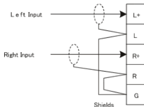
アンバランスステレオ音声の結線
