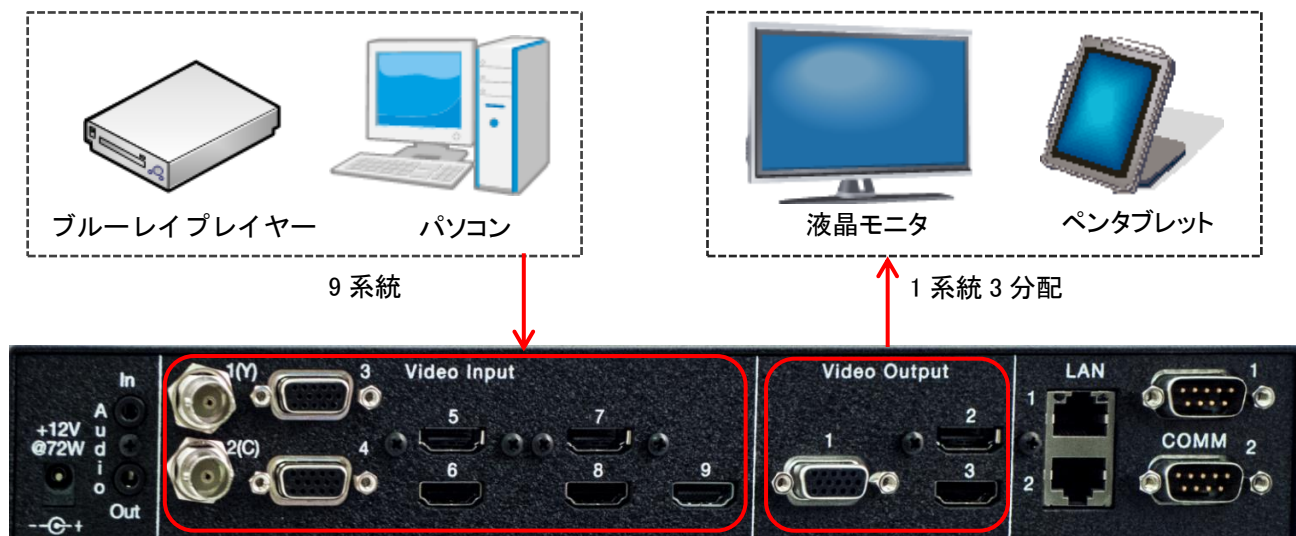
[図 5-1] ソース機器とシンク機器を接続したときの接続例
