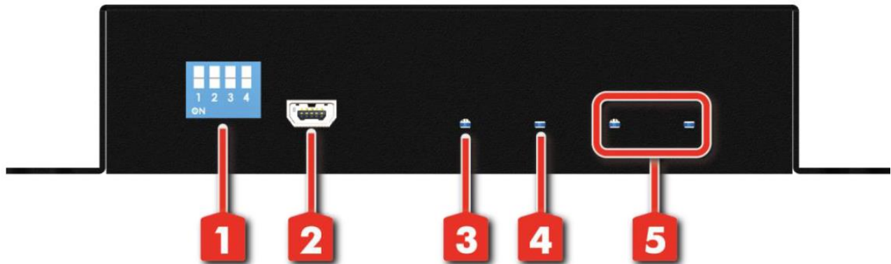
[図 3.1] フロントパネルの外観図
