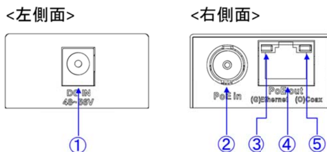
[図 4.2] 受信器(左右側面)
