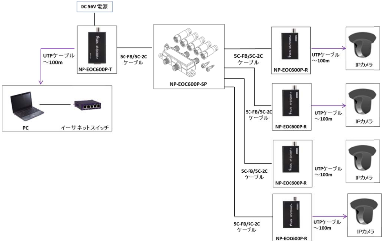
[図 5.5] 送信器と受信器の接続例
