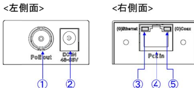
[図 4.1] 送信器(左右側面)
