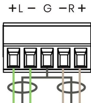
[図 4.3] 音声出力コネクタ—バランス結線図
