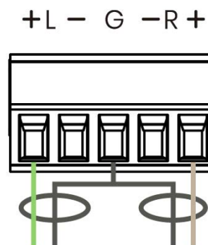
[図 4.4] 音声出力コネクタ—アンバランス結線図
