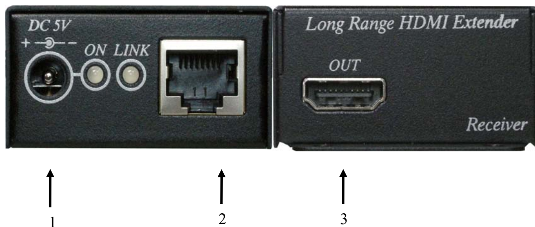
[図 1.2] 受信器パネル
