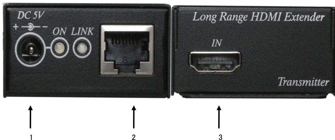
[図 1.1] 送信器パネル
