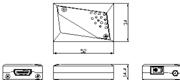
[図 6] 外形寸法図
