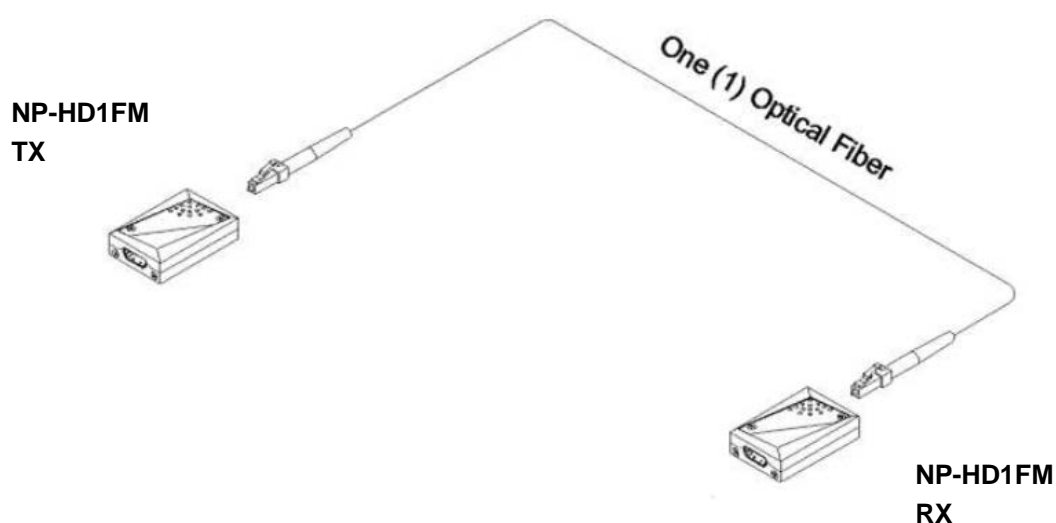
[図 3] モジュール間の光ファイバー接続
