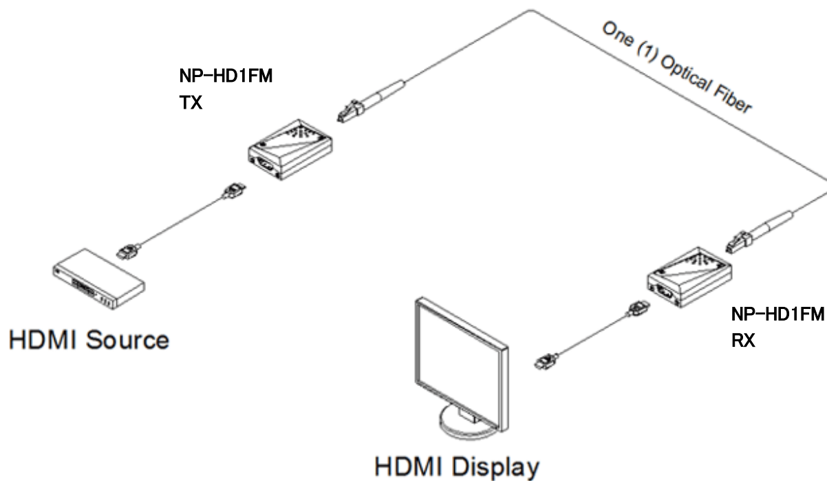
[図 1] HDMI 光延長着脱式モジュールの接続図
