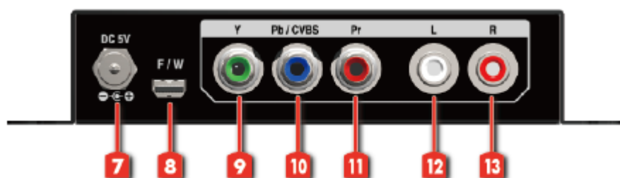
[図 3.2] リアパネルの外観図
