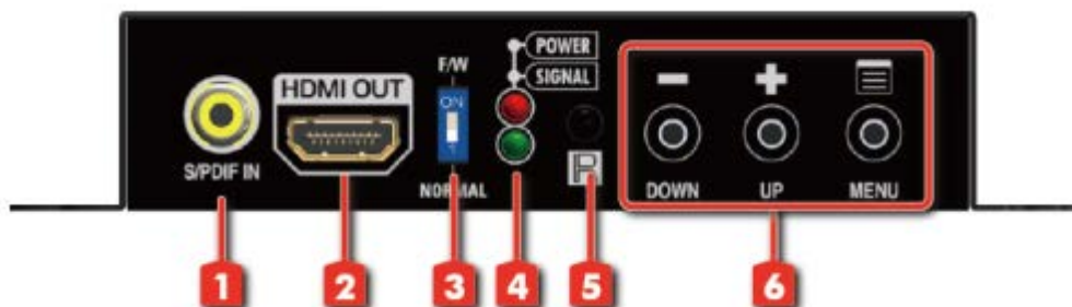
[図 3.1] フロントパネルの外観図
