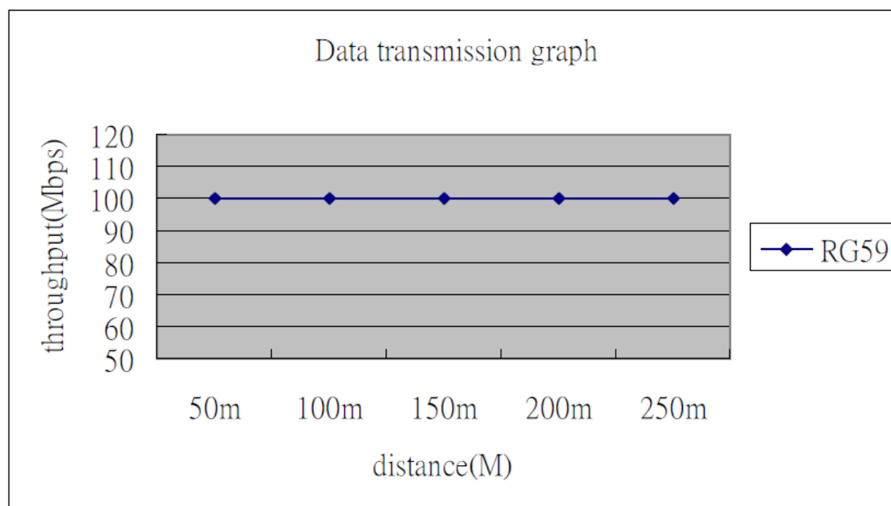
[表 6.3] 伝送距離の延長によるデータ損失(RG59 ケーブルの場合)
