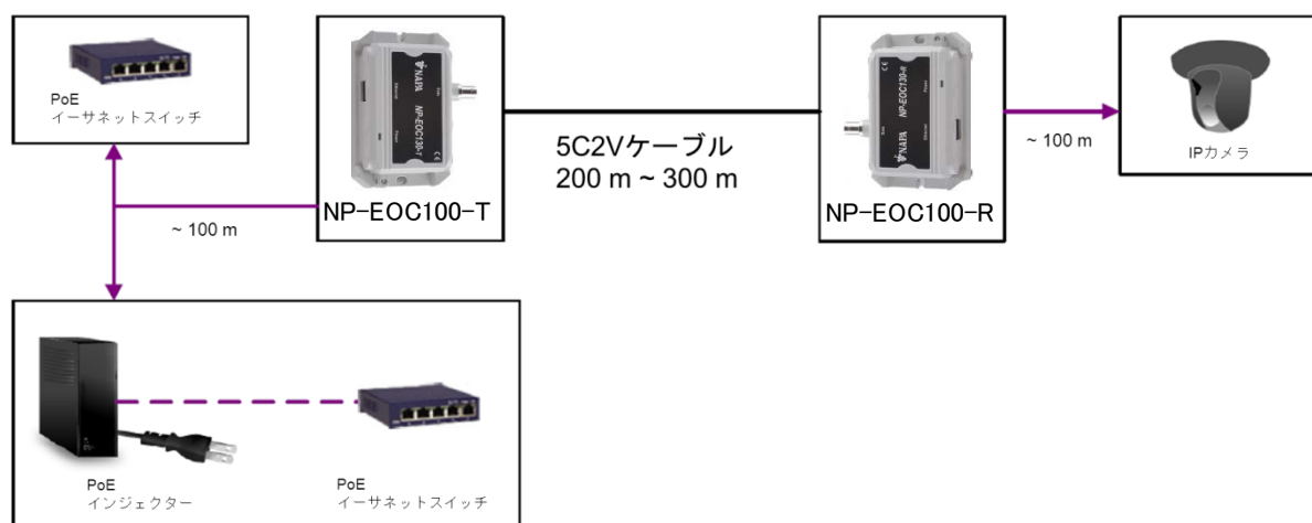
[図 4.1] NP-EOC100-TR 接続構成例
