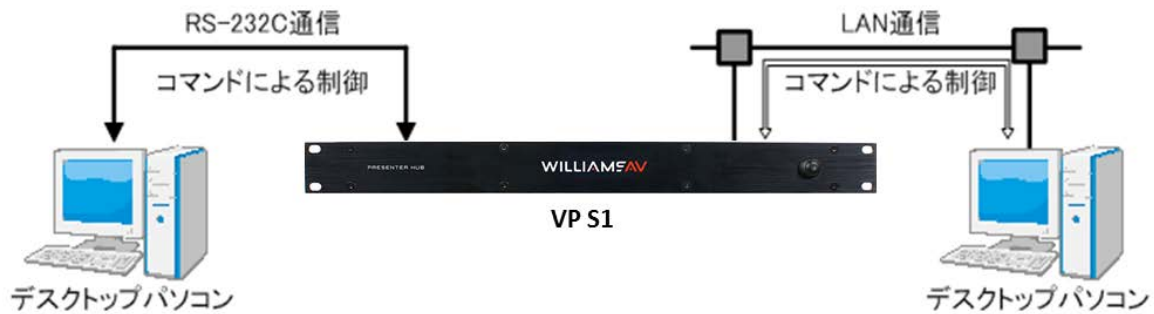
[図 1.1] 外部制御概要
